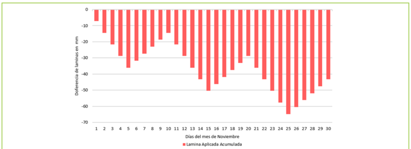
Figura 7: Diferencia entre lámina aplicada y lámina programada. Ejemplo práctico. Caudal solicitado de 400 l/s
