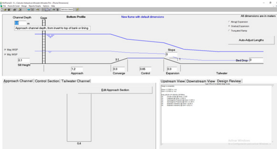
Figura 35: Ejemplo de aforador de cresta ancha- Modelo winflume
