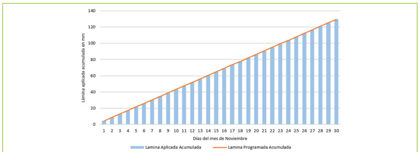
Figura 3: Lamina aplicada acumulada durante el mes. Ejemplo práctico. Canales A y B.
