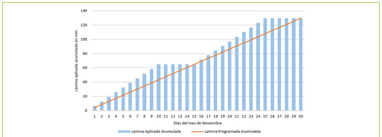
Figura 4: Lamina aplicada acumulada durante el mes de noviembre. Ejemplo práctico. Canal C.
