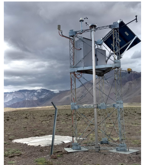
Figura 4. Estación Nivometeorológica del SIH-DGI.
