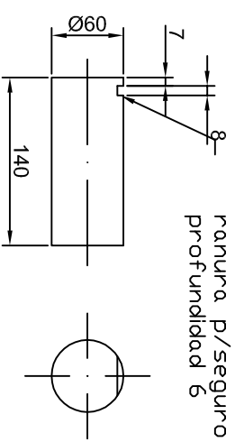
EJE DE RUEDA (Esc. 1:5) Material: Acero SAE 1045 c/baño de cromo esp. 0,3 Cantidad: 4 piezas
