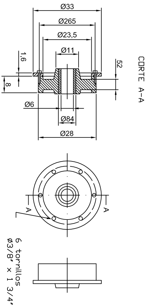
RUEDA CON PESTANA Material: Fundicion de hierro Buje: Grillon Poliamida 6 Cantidad: 4 piezas
