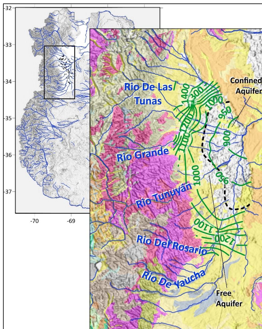
Figura 4-5: Niveles de agua subterránea (líneas verdes) en la cuenca central de Tunuyán Superior durante la temporada de invierno de 2022, contorneados en intervalos de 50 m 4 . Agua Superficial
