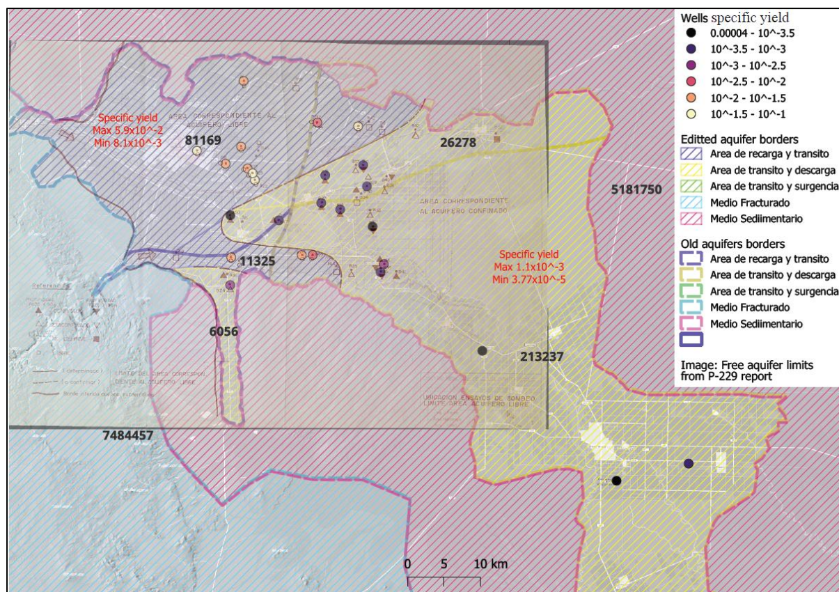
Figura 4-15: Rendimiento específico en la cuenca sur basado en datos de pruebas de bombeo de pozos (INA-CRAS, 1981), en comparación con las áreas de recarga administradas (ver también Figura 4-2 y línea gris en la Figura 4-14). Los rangos generalizados de rendimiento específico para cada área (compuestos por varios polígonos) se indican en rojo. Los números negros indican el área en hectáreas de cada polígono.
