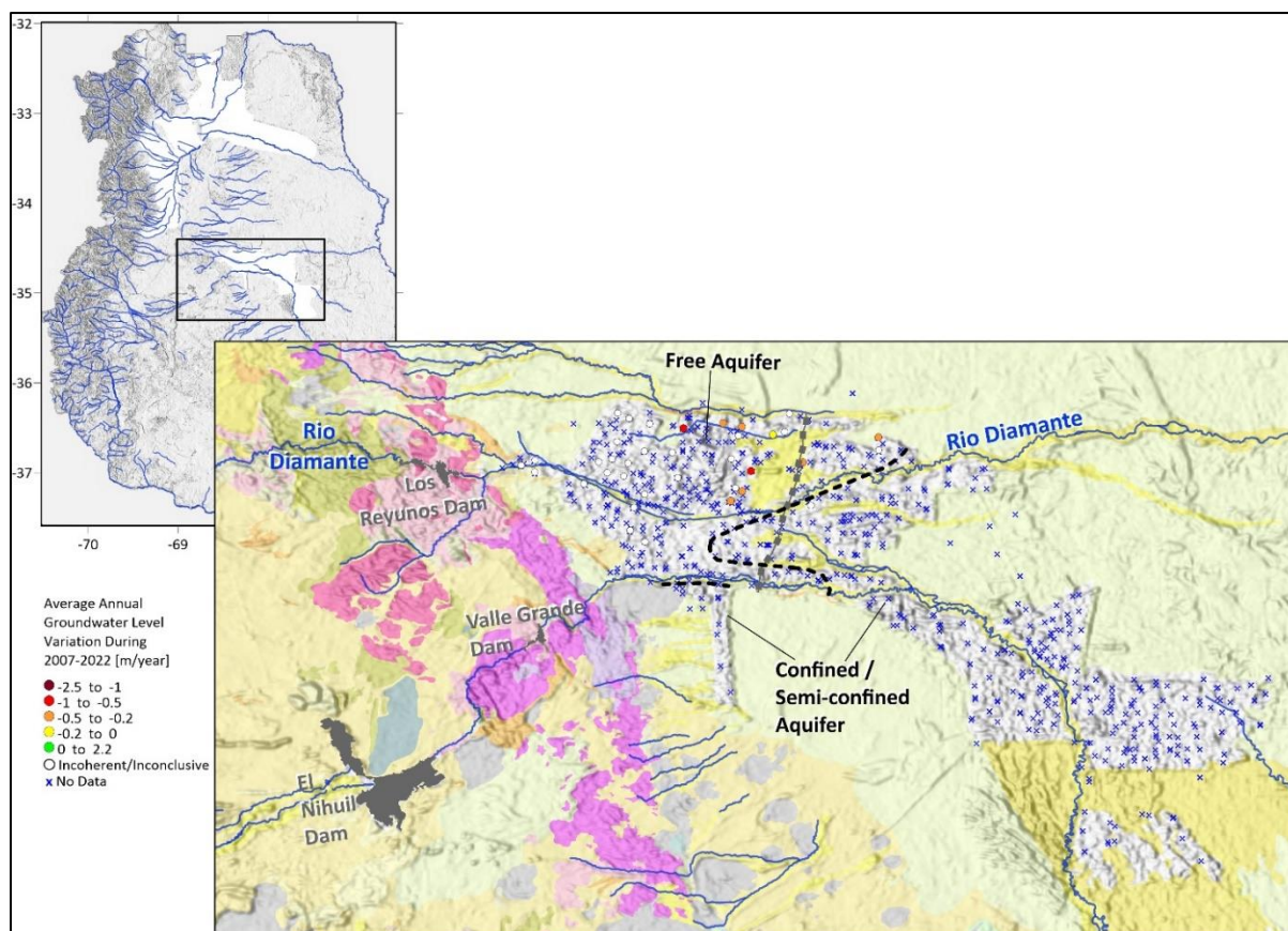
Figura 4-14. Variación promedio anual del nivel freático durante 2007-2022 en las zonas de recarga de la cuenca sur. 7
