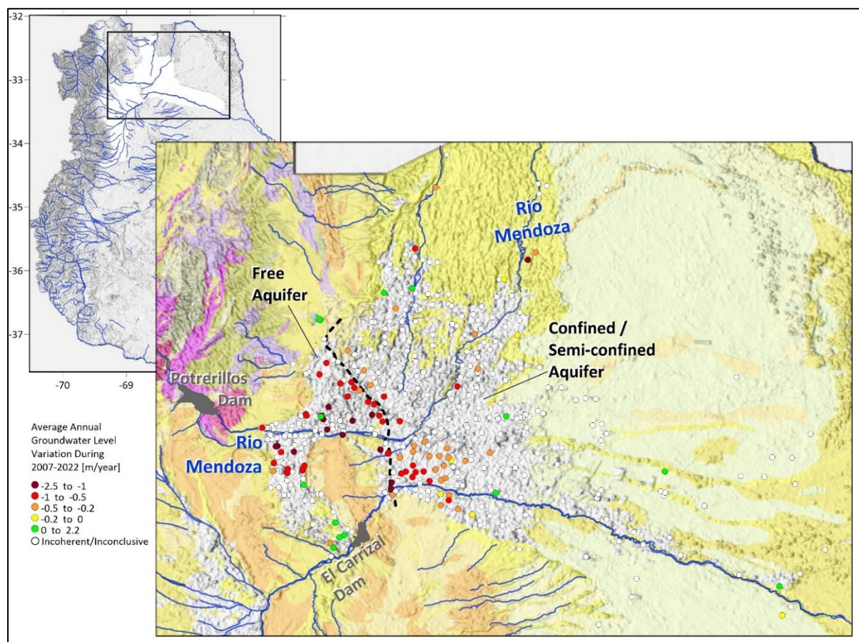
Figura 4-12: Variación promedio anual del nivel freático durante 2007-2022 en la cuenca norte. Se excluyen los pozos con coeficiente de correlación ( R^2 ) < 0,7 (círculos blancos).
