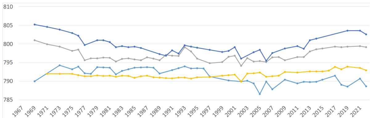
Figura 4-8: Hidrogramas de pozos seleccionados en el área de recarga de Margen Derecha de la cuenca norte. Se aprecia un aumento del nivel del agua subterránea durante 2007-2022.
