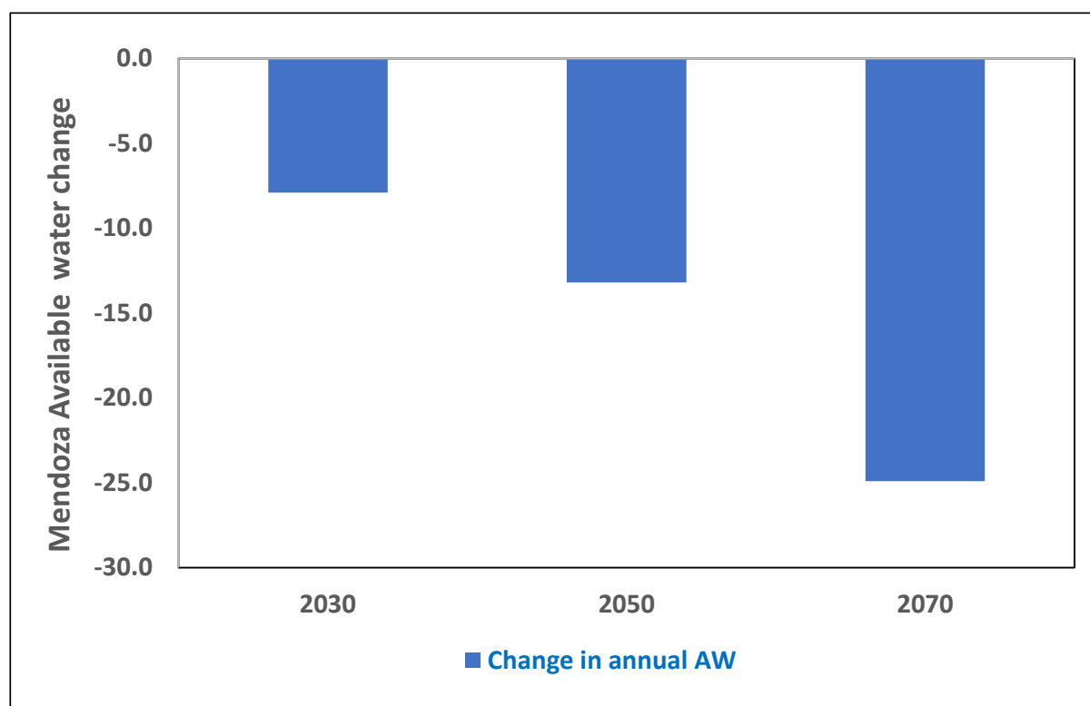
Figura 5-1: Cambios esperados (%) en los volúmenes de agua disponibles de Mendoza para los períodos 2030, 2050 y 2070 con respecto al período de referencia de 2000-2020
