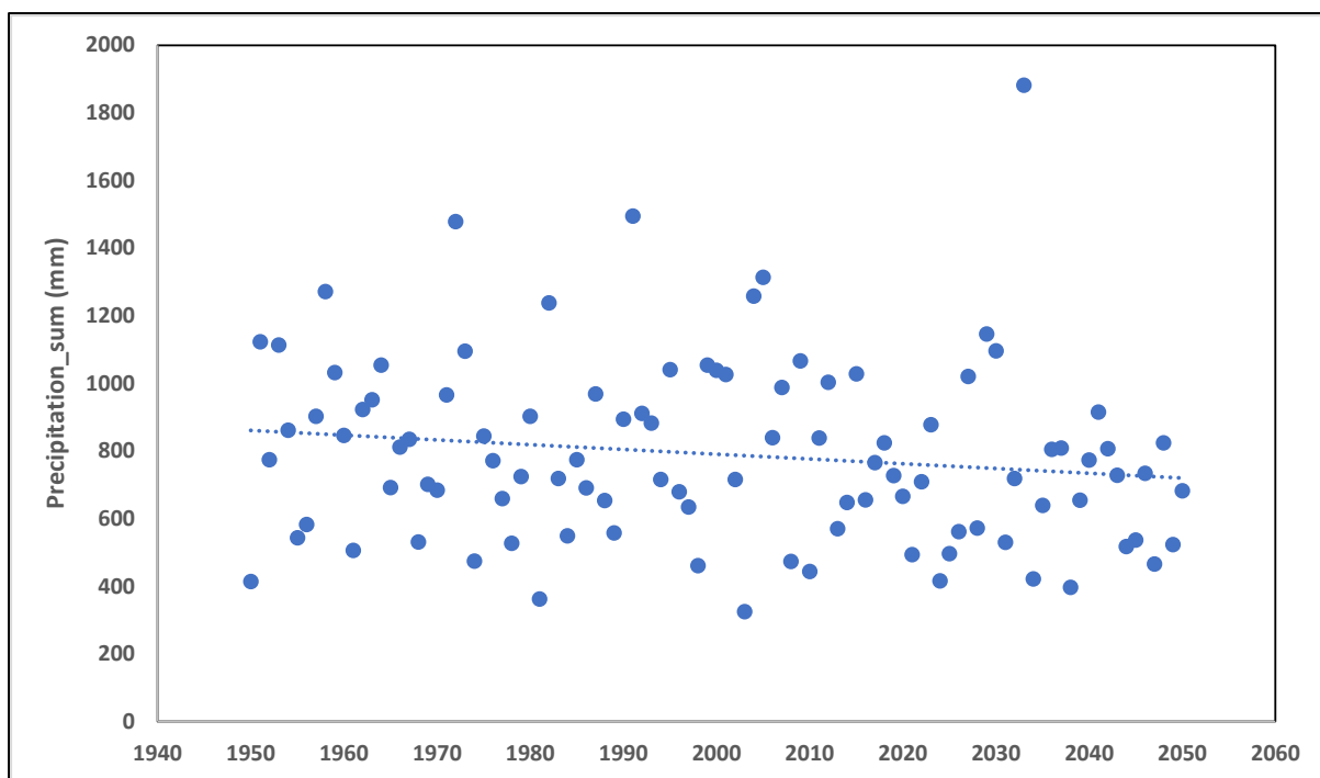
Figura 5-8: Precipitación anual simulada en las regiones andinas de gran altitud en Mendoza
