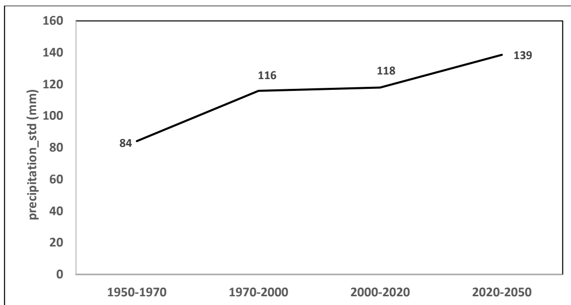
Figura 5-10: Desviación estándar de precipitación anual para Mendoza (regiones de gran altitud)
