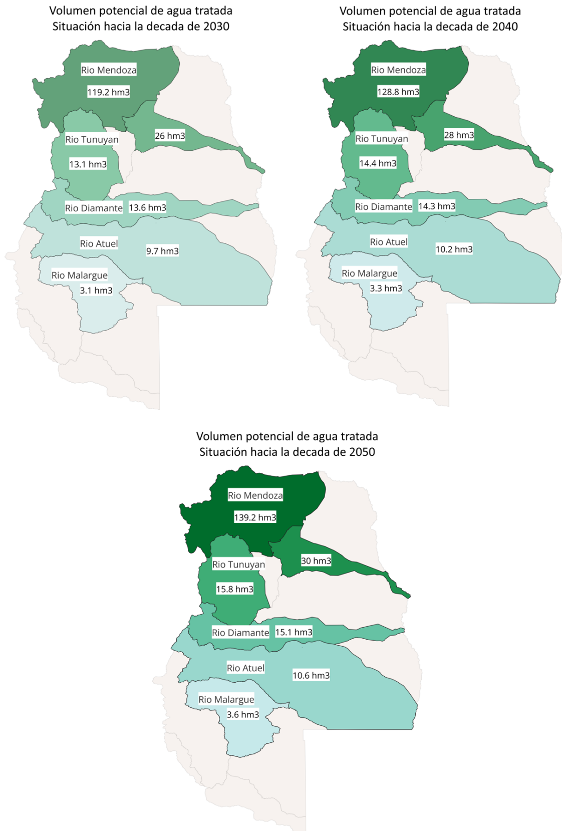
Figura 6-15: Volumen de agua tratada proyectado
