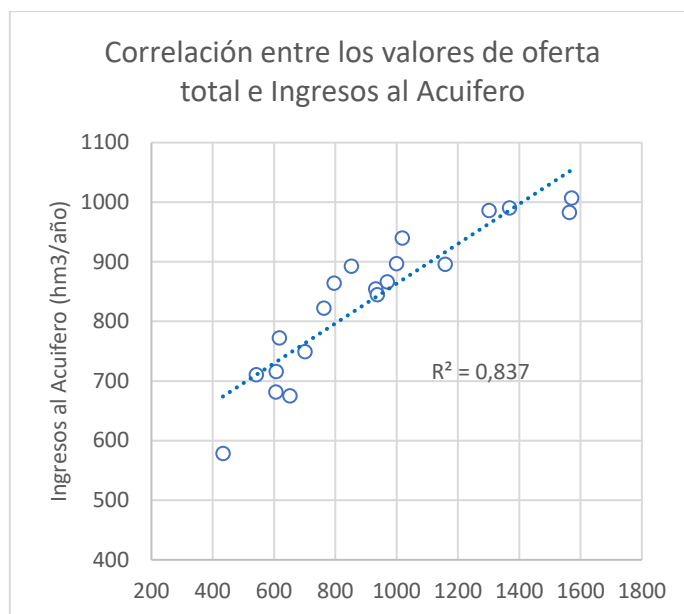
Figura 6-9: Correlación entre los valores de oferta total e Ingresos al acuífero (Atuel)
