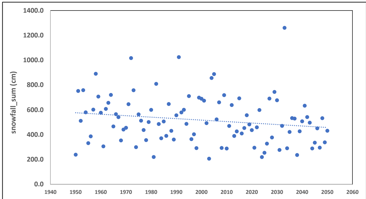
Figura 5-12: Acumulación anual de nieve en la zona de los Andes de Mendoza: 5126m
