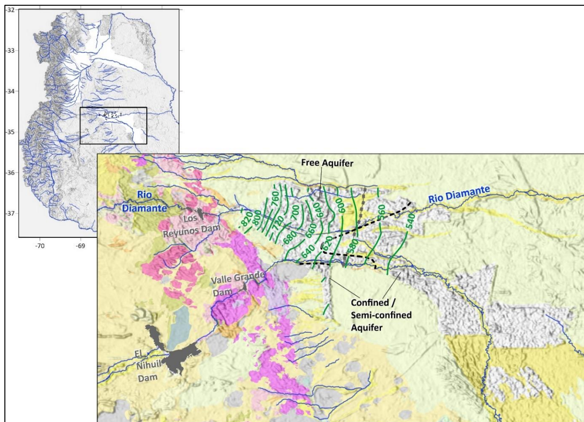
Figura 4-6. Niveles freáticos (líneas verdes) en las zonas Diamante y Atuel de la cuenca sur durante la temporada invernal de 2022, contorneados en intervalos de 20 m. 5
