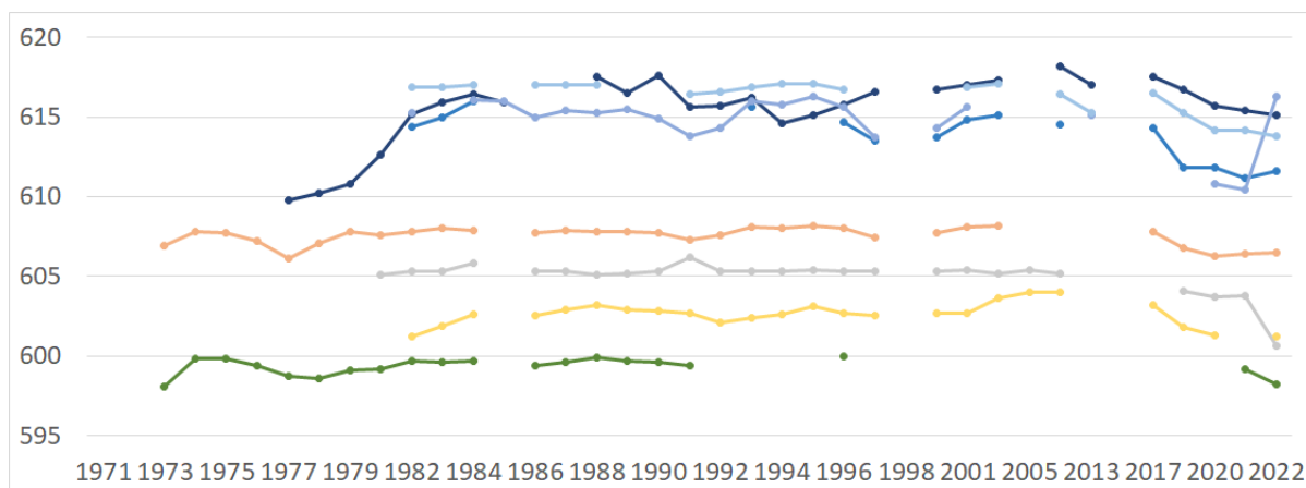
Figura 4-11: Hidrogramas de pozos seleccionados en las zonas de recarga de la Cuenca Sur. La falta de datos aumenta la incertidumbre de las tendencias de los niveles de agua subterránea.
