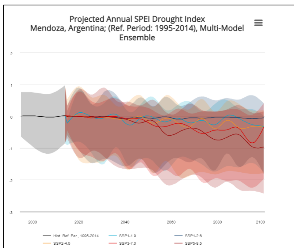
Figura 5-11: El índice de sequía SPEI (precipitación y evaporación) para diferentes escenarios climáticos para Mendoza
