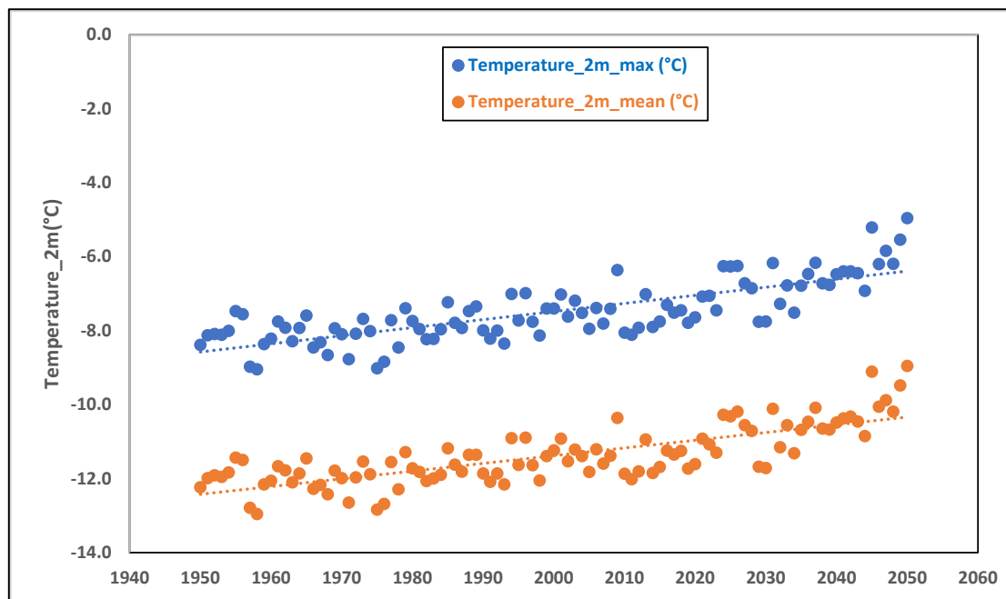
Figura 5-5: Media (naranja) y máx. (azul) tendencia de las temperaturas anuales en los Andes de Mendoza, 5126 m
