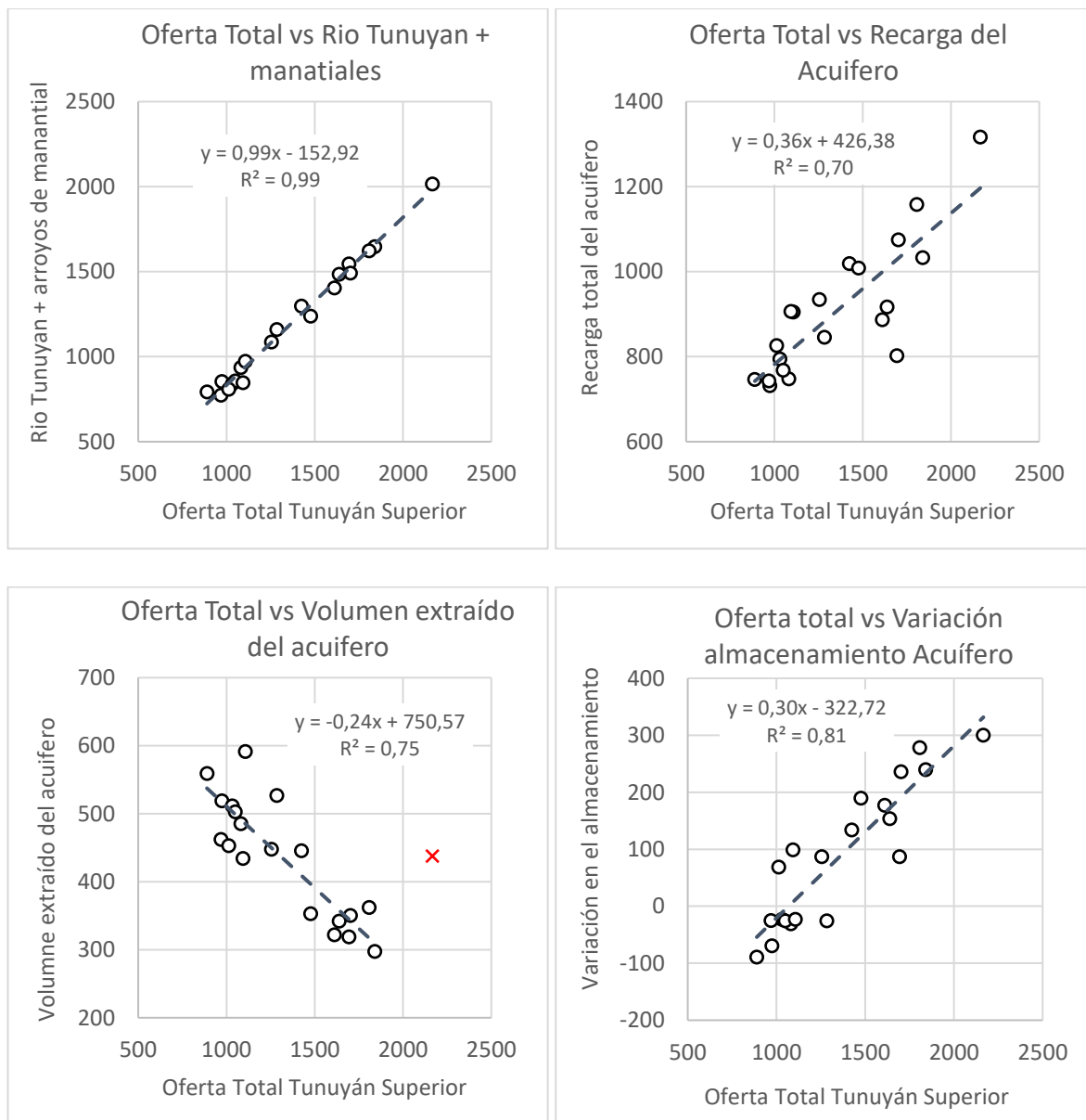
Figura 6-1: Correlaciones entre las distintas variables
