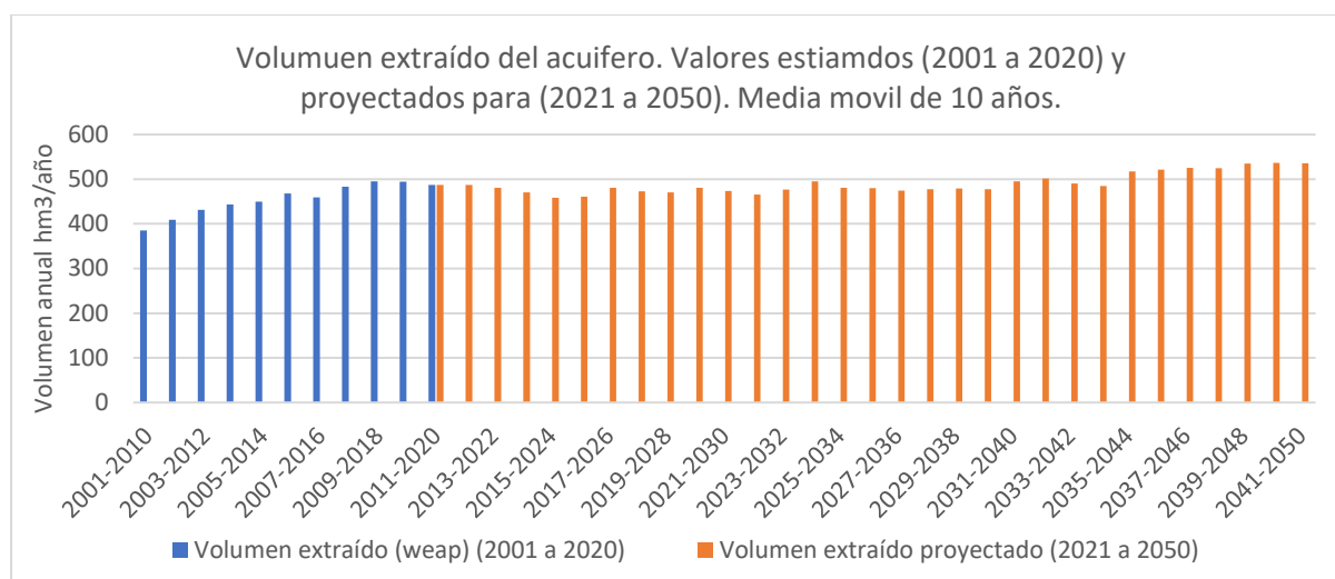
Figura 6-7: Media móvil de 10 años. Volumen Extraído del acuífero, escenario proyectado a 2050
