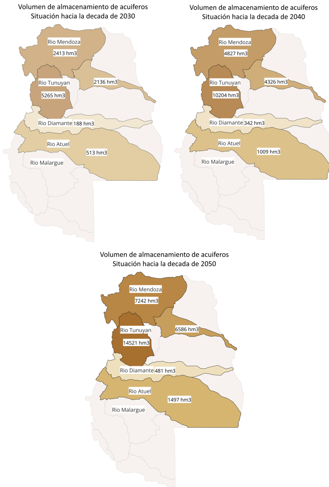
Figura 6-14: Volumen Acumulado De Agua Subterránea Proyectado
