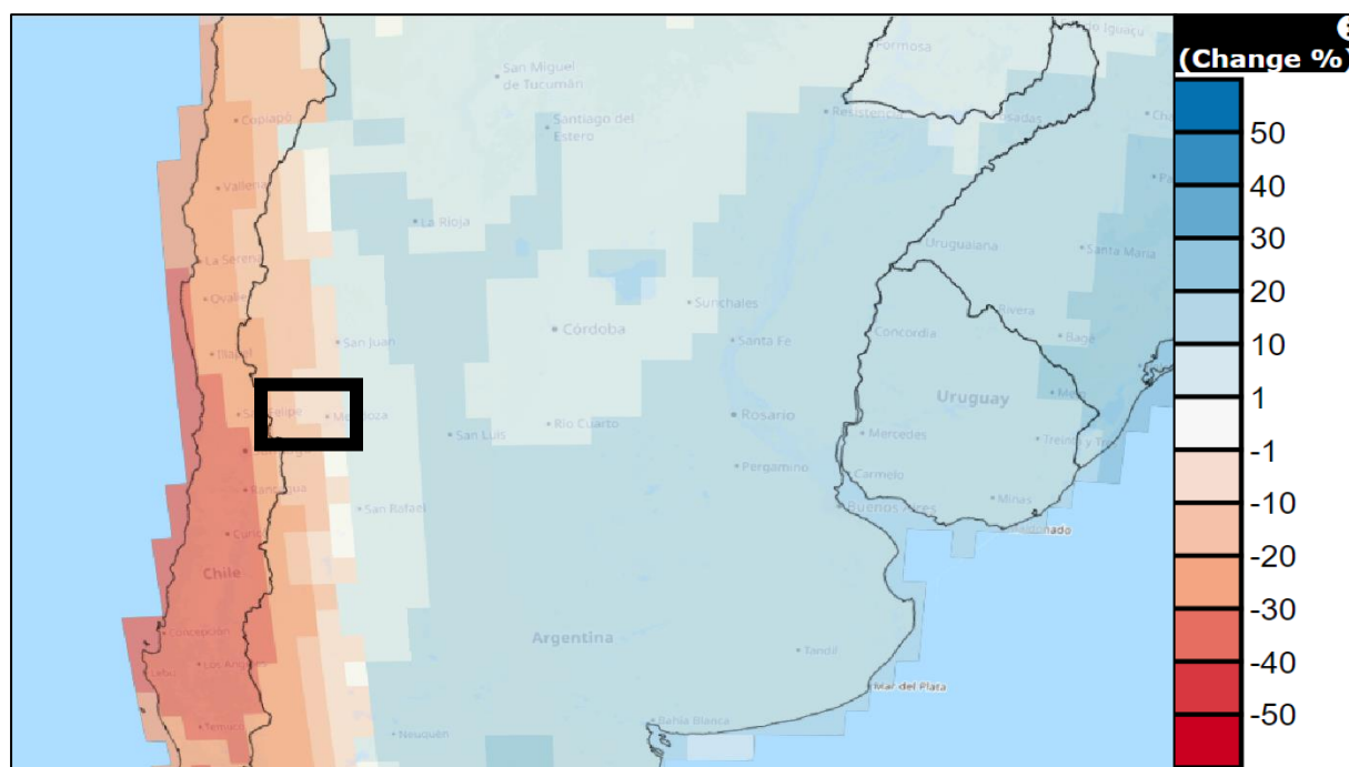
Figura 5-7: Anomalía de precipitación (%) para el período 2030 - 2050 con respecto a la línea base 1970-2000.
