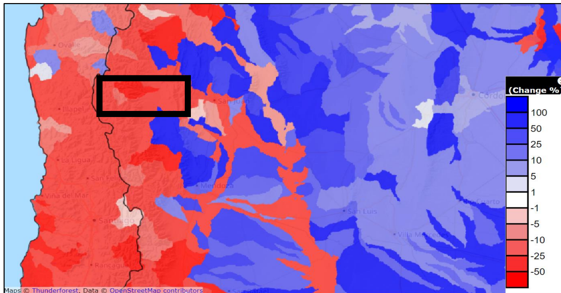
Figura 5-13: Anomalía del volumen medio anual de caudales para el período 2030-2050 con respecto a la línea base 1970-2000
