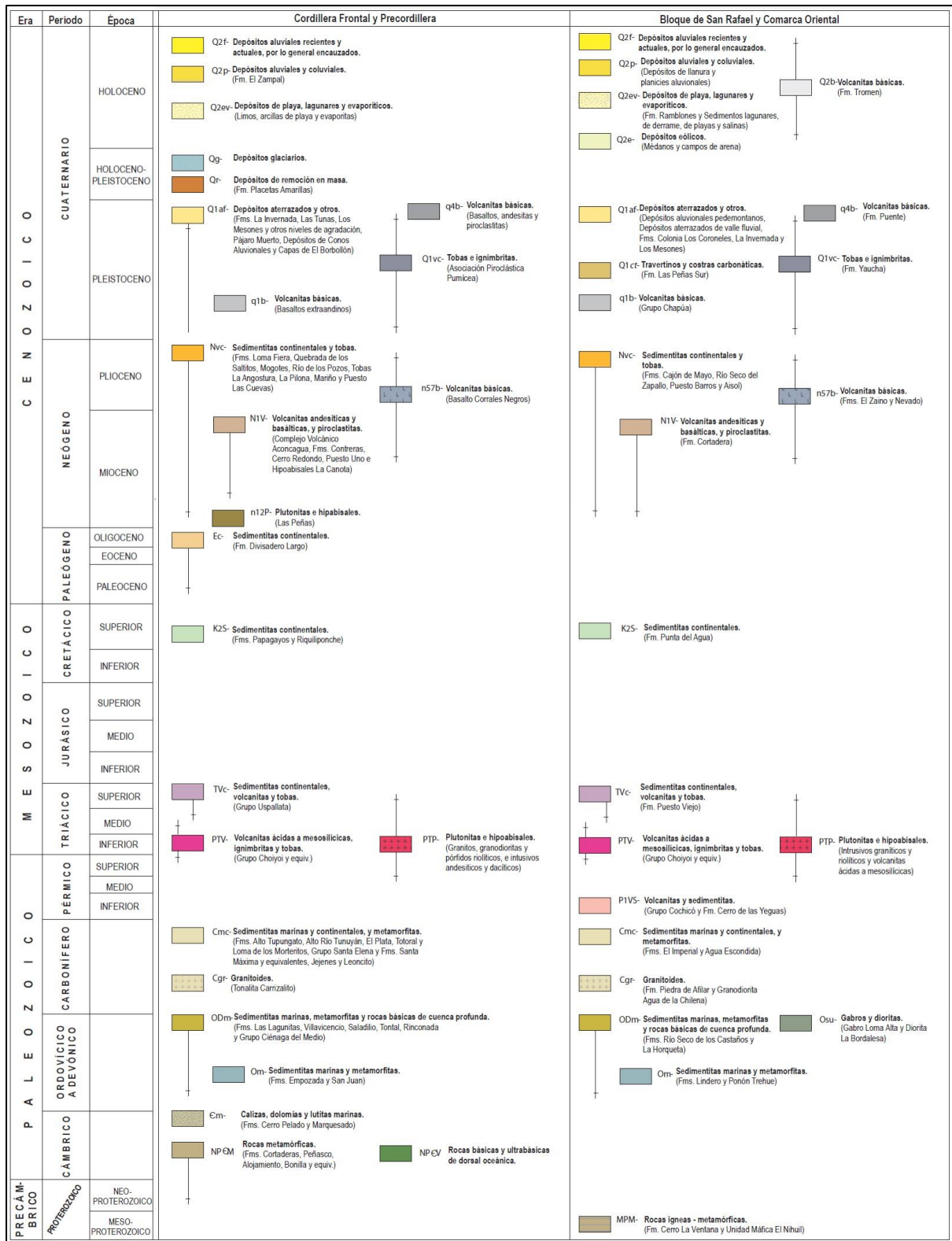
Figura 4-3: Columna estratigráfica de la provincia de Mendoza. Los colores corresponden al mapa geológico de la Figura 4-2.
