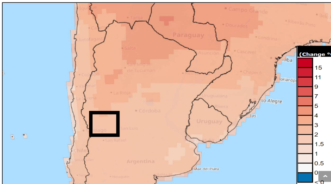
Figura 5-4: Anomalía de las temperaturas medias para el periodo 2020-2040 respecto a la línea base
