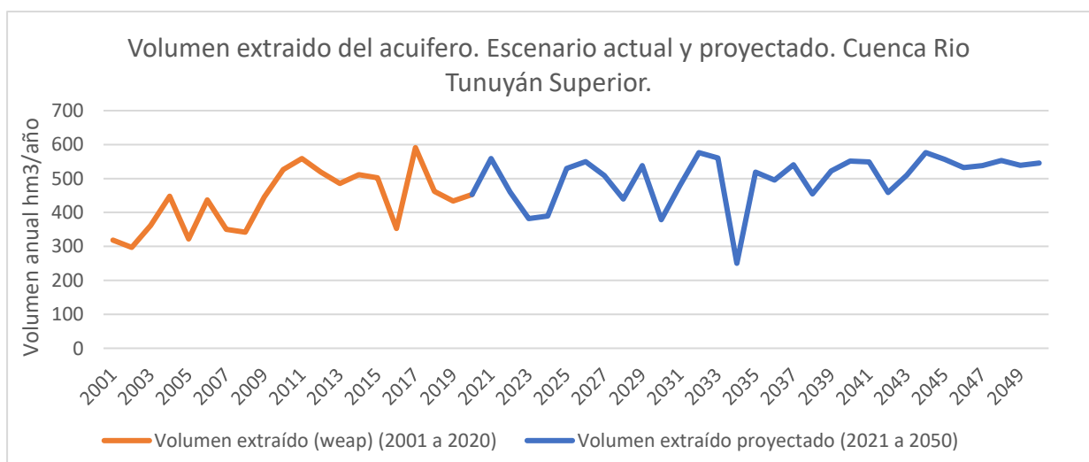
Figura 6-6: Volumen extraído del acuífero, proyectado al año 2050
