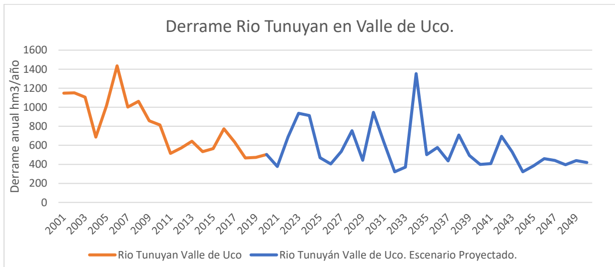
Figura 6-5: Derrames anuales Río Tunuyán en Valle de Uco hacia el año 2050
