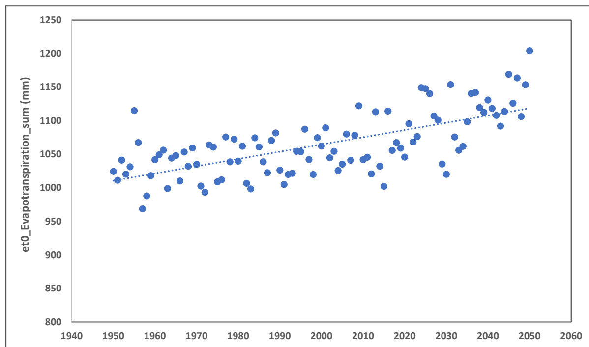
Figura 5-6: Evaporación anual en Mendoza, elevación 1665 m
