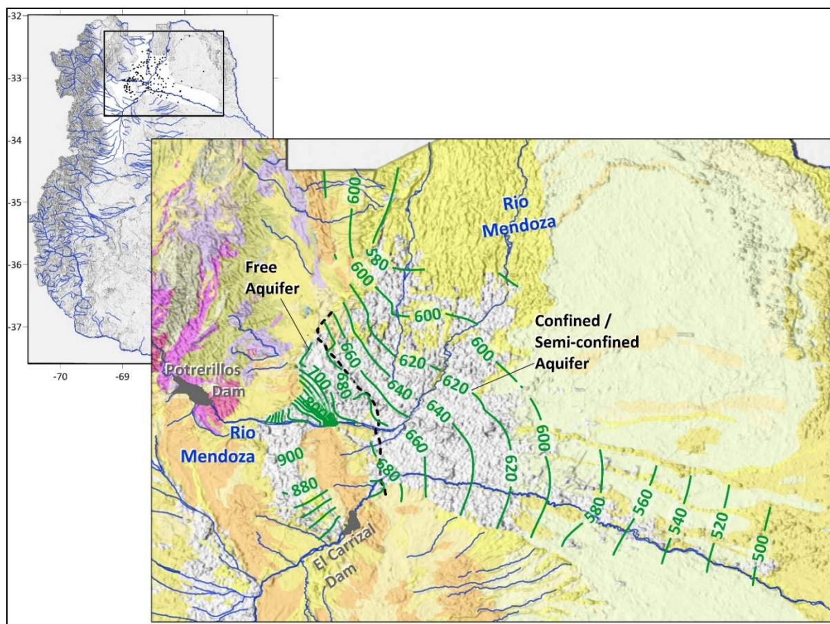
Figura 4-4: Niveles de agua subterránea (líneas verdes) en la cuenca norte durante la temporada de invierno de 2022, perfilados en intervalos de 20 m 3 .
