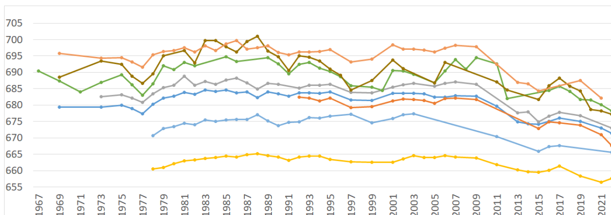
Figura 4-9: Hidrogramas de pozos seleccionados en el área de recarga Tunuyán Inferior de la cuenca norte. Se aprecia una disminución del nivel del agua subterránea durante 2007-2022.
