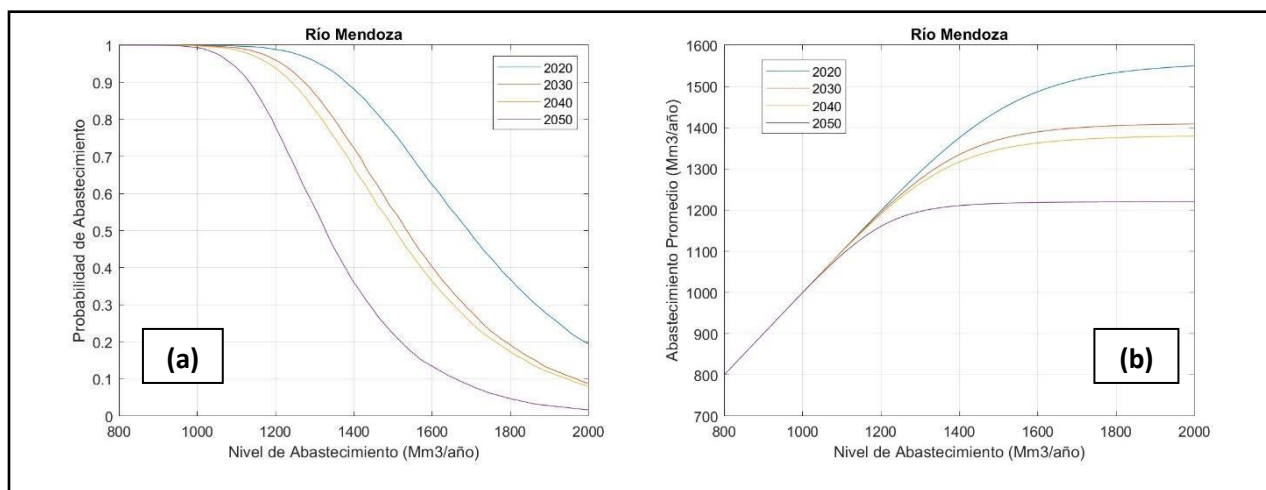
Figura 5-8: Río Mendoza variación de, (a) Probabilidad de Abastecimiento y (b) Abastecimiento Promedio, para distintos Niveles de Abastecimiento y Capacidad de Almacenamiento Fija que duplica la existente (800 Mm 3 ) para 2020, 2030, 2040 y 2050.
