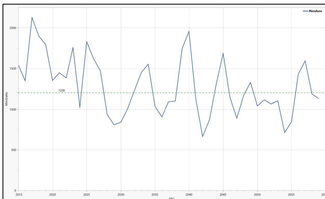
Figura 5-3: Proyección de caudales anuales en el río Mendoza y nivel de abastecimiento de 1200 Mm 3 /año.
