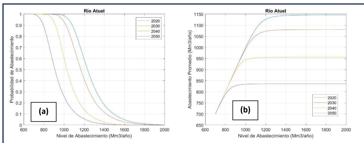
Figura 5-12: Río Atuel variación de, (a) Probabilidad de Abastecimiento y (b) Abastecimiento Promedio, para distintos Niveles de Abastecimiento y Capacidad de Almacenamiento Fija que duplica la existente (700 Mm 3 ) para 2020, 2030, 2040 y 2050.
