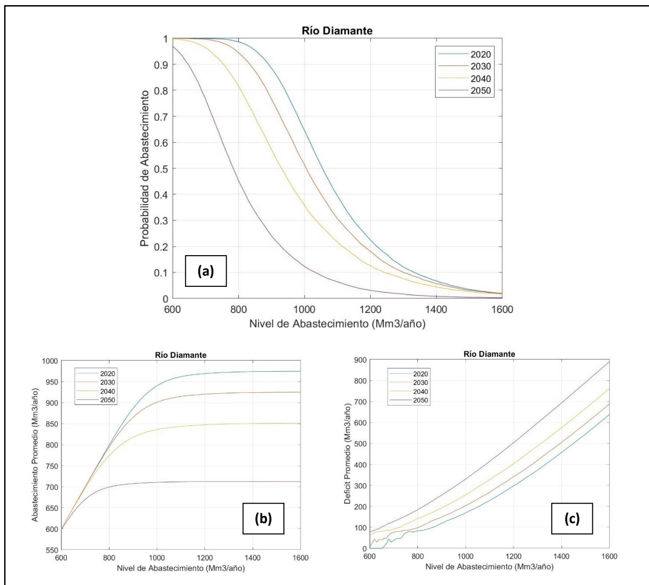
Figura 5-13: Río Diamante variación de, (a) Probabilidad de Abastecimiento, (b) Abastecimiento Promedio y (c) Déficit Promedio, para distintos Niveles de Abastecimiento y Capacidad de Almacenamiento Fija (544 Mm 3 ) para 2020, 2030, 2040 y 2050.
