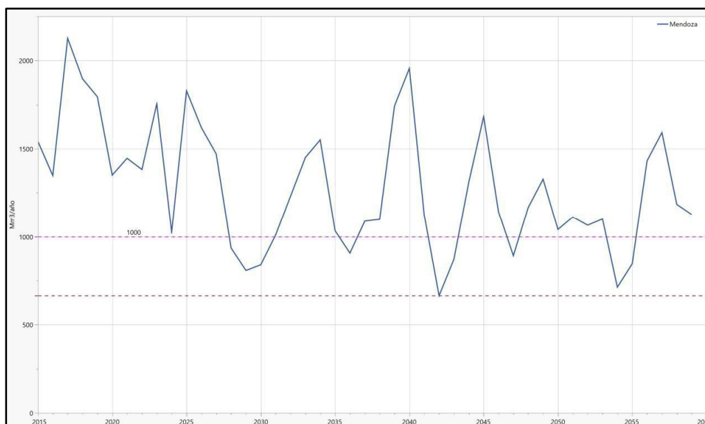
Figura 5-1: Proyección de caudales anuales en el río Mendoza
