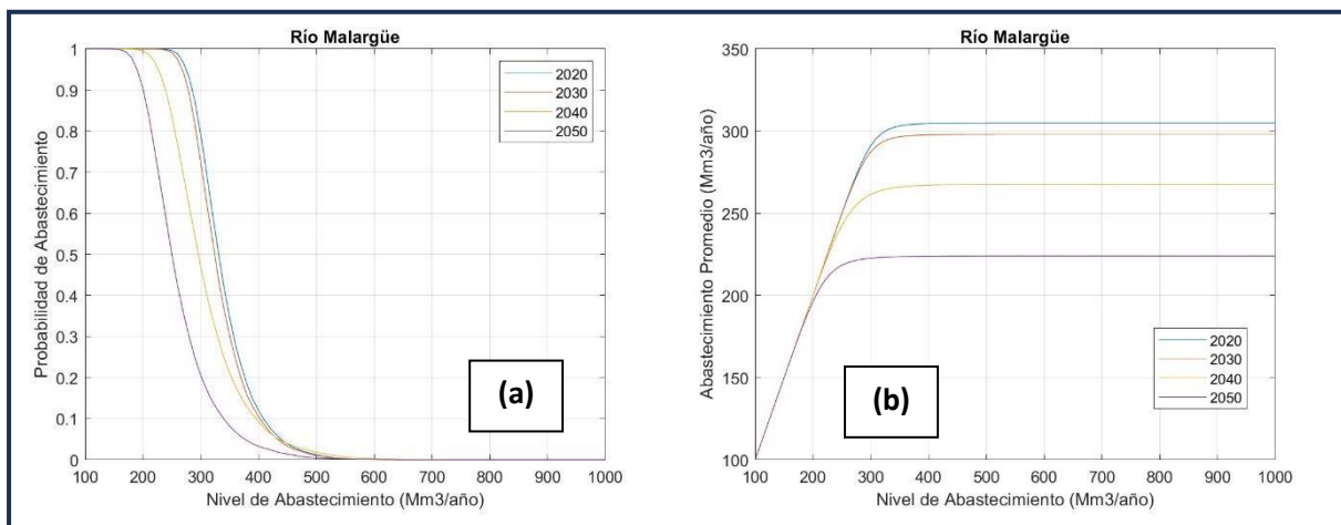
Figura 5-15: Río Malargüe variación de, (a) Probabilidad de Abastecimiento, (b) Abastecimiento Promedio y (c) Déficit Promedio, para distintos Niveles de Abastecimiento y Capacidad de Almacenamiento Fija (0 Mm 3 ) para 2020, 2030, 2040 y 2050.
