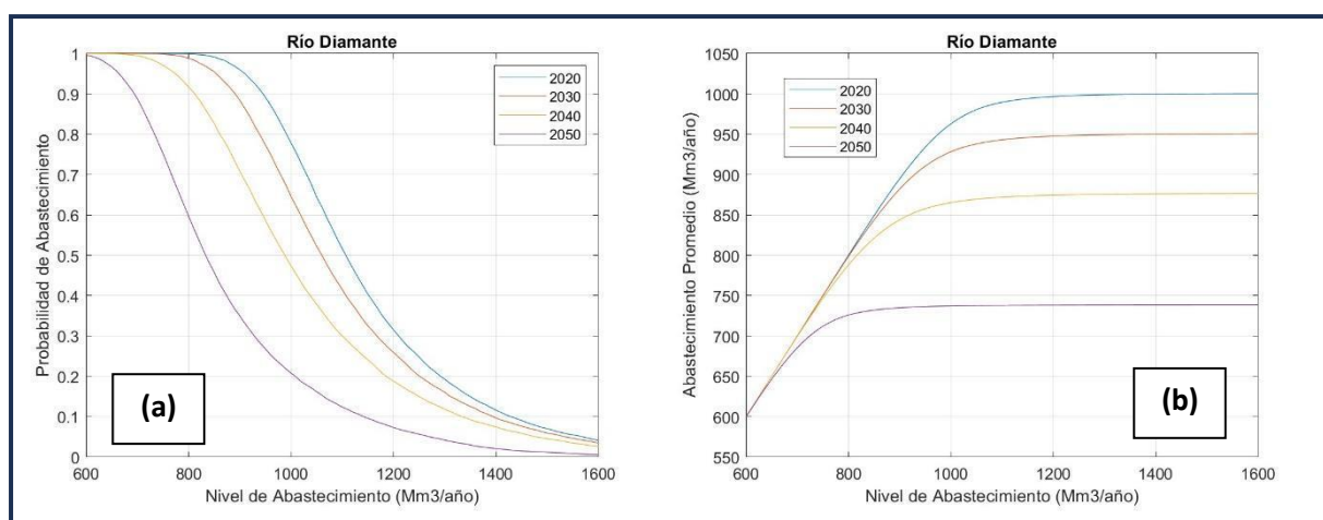
Figura 5-14: Río Diamante variación de, (a) Probabilidad de Abastecimiento y (b) Abastecimiento Promedio, para distintos Niveles de Abastecimiento y Capacidad de Almacenamiento Fija que duplica la existente (1100 Mm 3 ) para 2020, 2030, 2040 y 2050.
