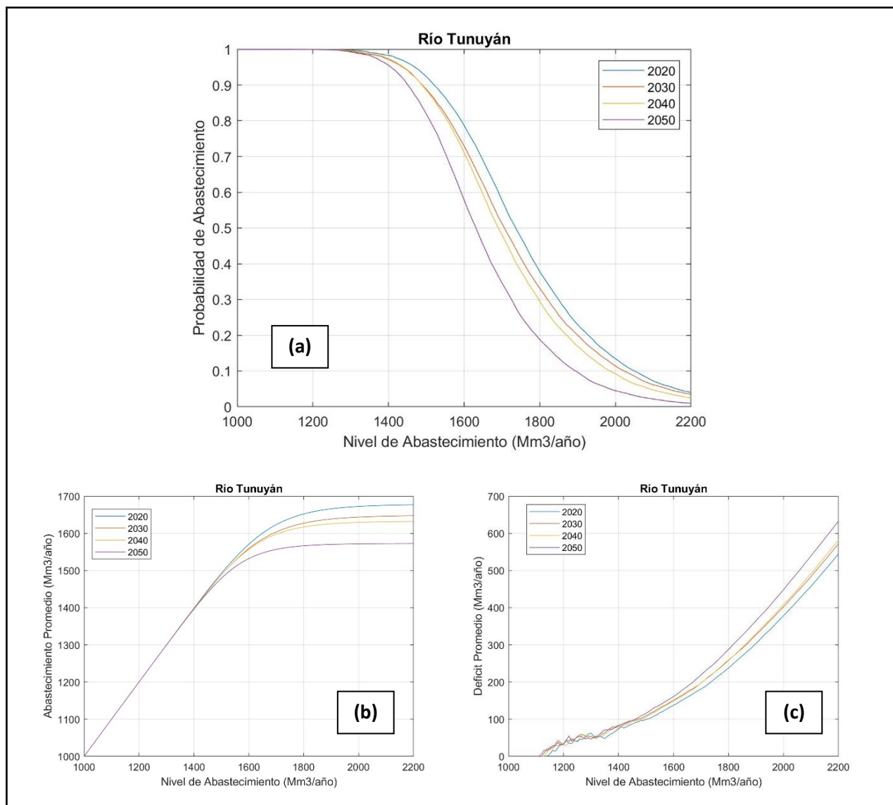
Figura 5-9: Río Tunuyán variación de, (a) Probabilidad de Abastecimiento, (b) Abastecimiento Promedio y (c) Déficit Promedio, para distintos Niveles de Abastecimiento y Capacidad de Almacenamiento Fija (276 Mm 3 ) para 2020, 2030, 2040 y 2050.
