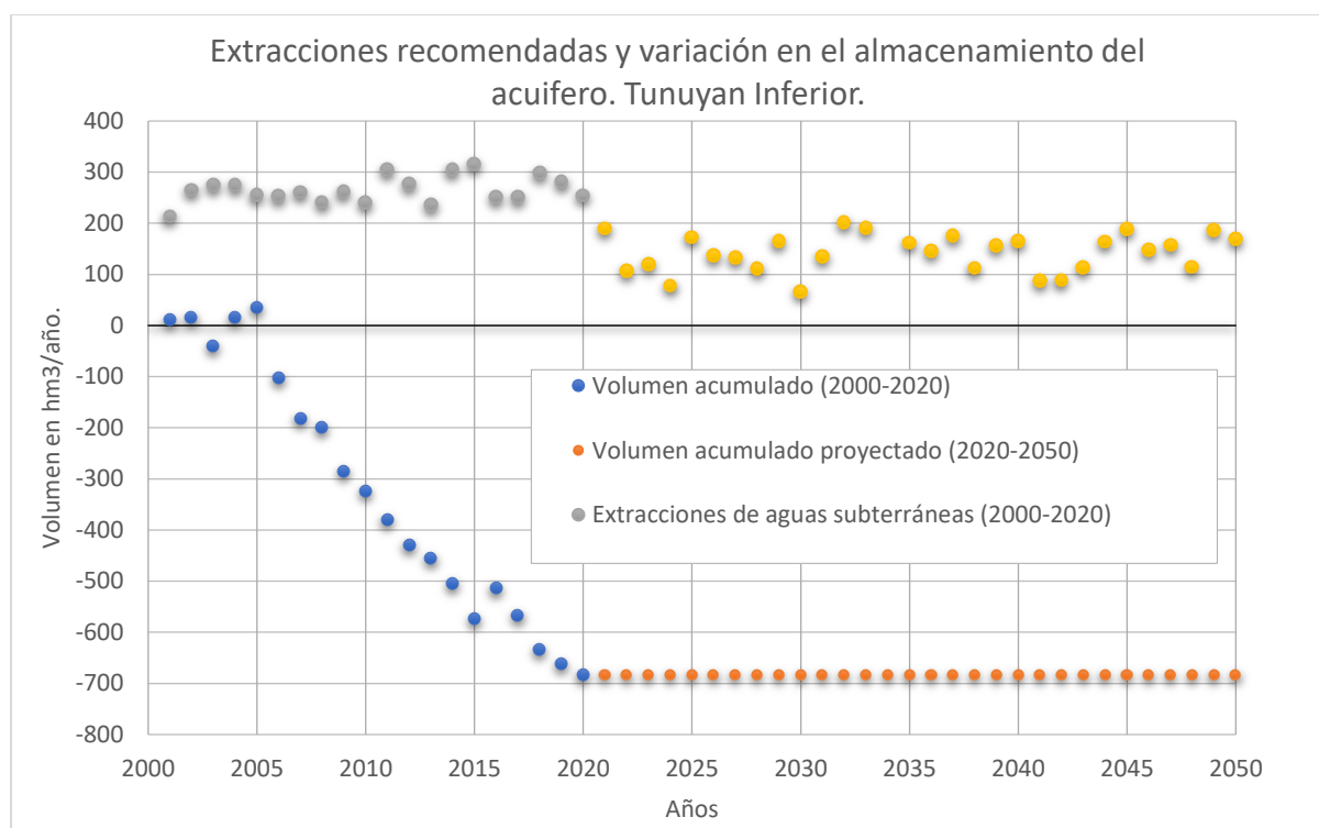
Figura 4-1: Extracciones recomendadas y variación en el almacenamiento del acuífero. Tunuyan Inferior
