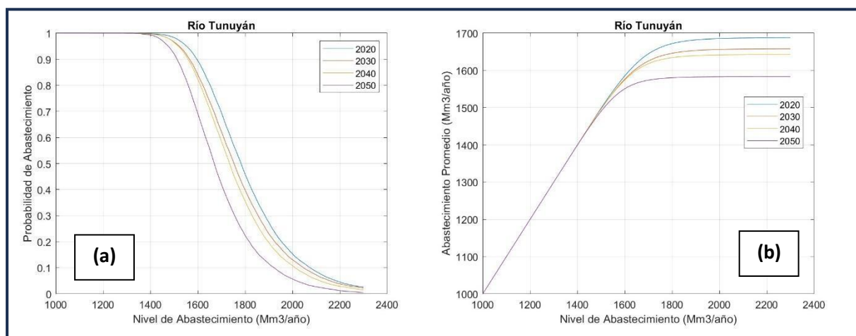
Figura 5-10: Río Tunuyán variación de, (a) Probabilidad de Abastecimiento y (b) Abastecimiento Promedio, para distintos Niveles de Abastecimiento y Capacidad de Almacenamiento Fija que duplica la existente (600 Mm 3 ) para 2020, 2030, 2040 y 2050.
