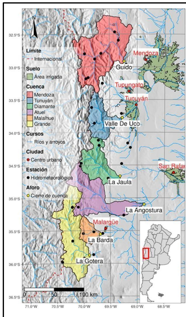
Figura 5-5: Cuencas hídricas usadas para la modelización hidrológica con HBV.IANIGLA. Se marcan los puntos de cierre de estas (círculos amarillos) y las estaciones hidrometeorológicas analizadas y procesadas (círculos negros). (IANIGLA, 2023).
