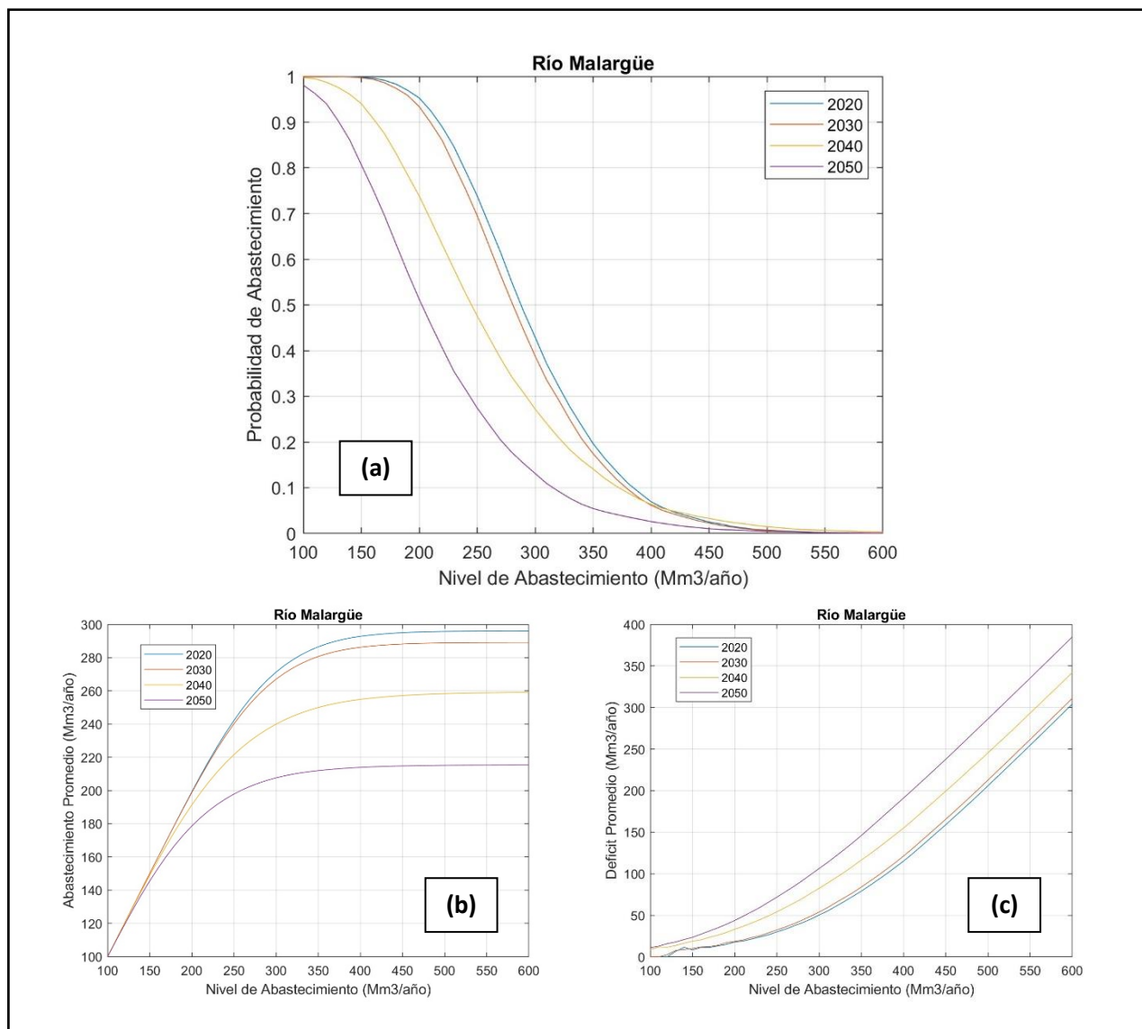
Figura 5-15: Río Malargüe variación de, (a) Probabilidad de Abastecimiento, (b) Abastecimiento Promedio y (c) Déficit Promedio, para distintos Niveles de Abastecimiento y Capacidad de Almacenamiento Fija (0 Mm 3 ) para 2020, 2030, 2040 y 2050.
