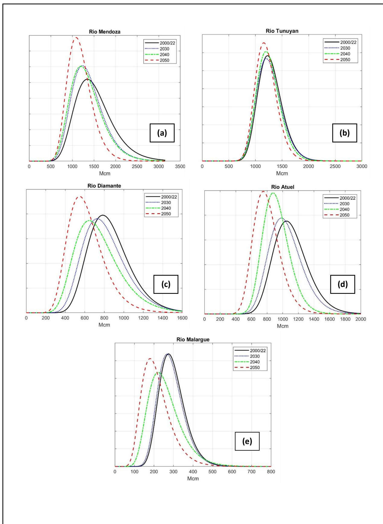
Figura 5-6: Distribución actual (2020) y de la proyección de los caudales anuales en los ríos (a) Mendoza, (b) Tunuyán, (c) Diamante, (d) Atuel y (e) Malargüe para 2030, 2040 y 2050.
