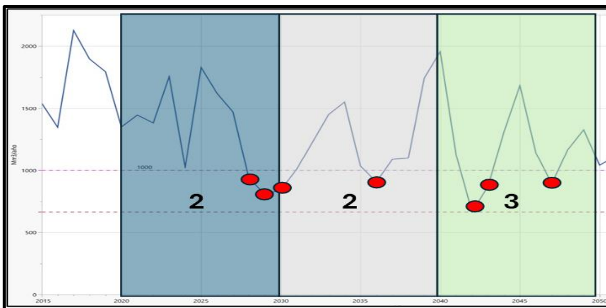
Figura 5-2: Proyección de caudales anuales en el río Mendoza y confiabilidad para un nivel de abastecimiento de 1.000 Mm 3 por año.
