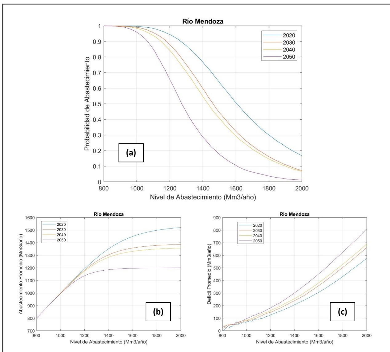
Figura 5-7: Río Mendoza variación de, (a) Probabilidad de Abastecimiento, (b) Abastecimiento Promedio y (c) Déficit Promedio, para distintos Niveles de Abastecimiento y Capacidad de Almacenamiento Fija (395 Mm 3 ) para 2020, 2030, 2040 y 2050.
