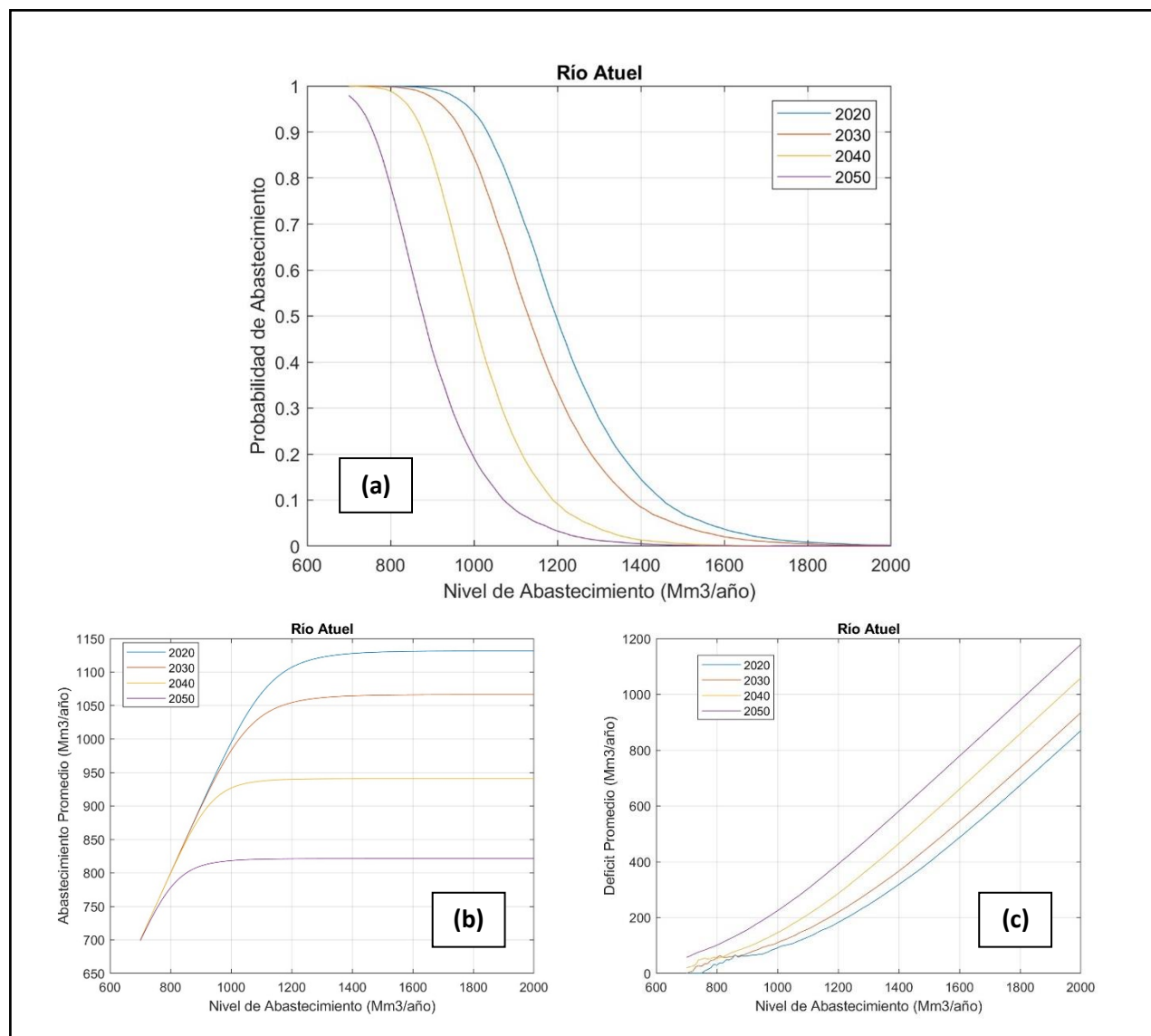
Figura 5-11: Río Atuel variación de, (a) Probabilidad de Abastecimiento, (b) Abastecimiento Promedio y (c) Déficit Promedio, para distintos Niveles de Abastecimiento y Capacidad de Almacenamiento Fija (352 Mm 3 ) para 2020, 2030, 2040 y 2050.
