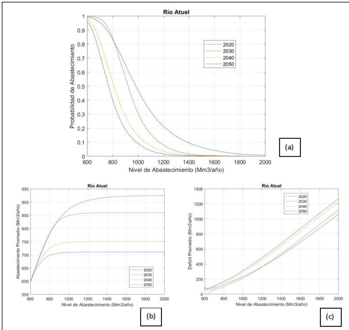
Figura 2.3: Río Atuel variación de, (a) Probabilidad de Abastecimiento, (b) Abastecimiento Promedio y (c) Déficit Promedio, para distintos Niveles de Abastecimiento y Capacidad de Almacenamiento Fija (352 Mm 3 ) para 2020, 2030, 2040 y 2050.
