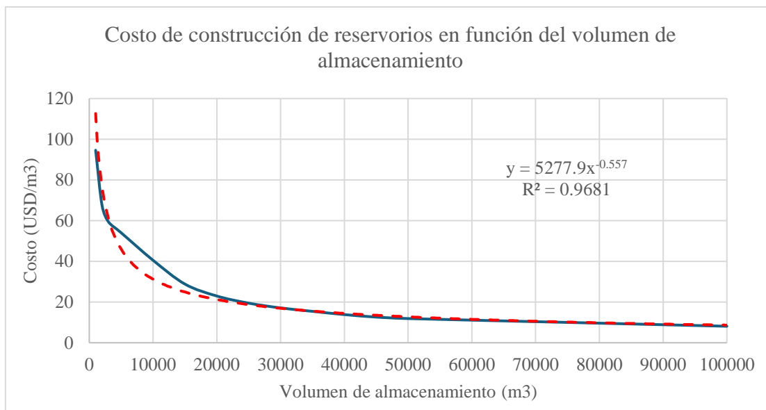
Figura 8.1: Costo de construcción de reservorios Fuente: Compañía nacional de agua de Israel.
