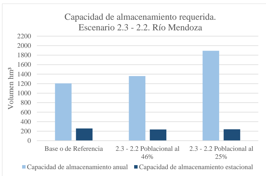
Figura 9.3: Capacidad de almacenamiento requerida. Escenario 2.3 – 2.2. Cuenca del Mendoza.
