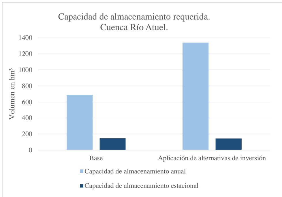
Figura 9.11: Capacidad de almacenamiento requerida. Cuenca del Río Atuel.
