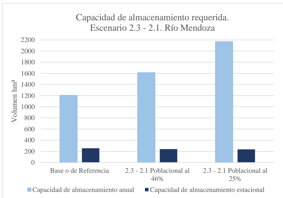
Figura 9.4: Capacidad de almacenamiento requerida. Escenario 2.3 – 2.1. Cuenca del Mendoza.
